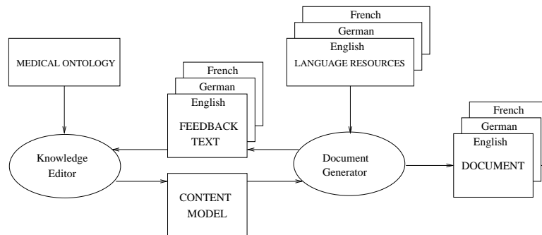
Figure 2: WYSIWYM editing
