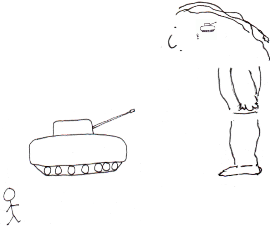
Figure 1: Ambush scenario.
